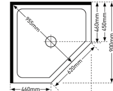
ANGLED 900 X 900
